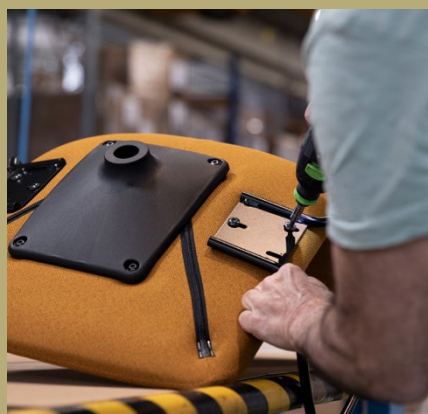
Après avoir percé le tissu, les accessoires mécaniques du piétement peuvent être fixés. L'assemblage est manuel et le contrôle des pièces avant livraison est visuel.
